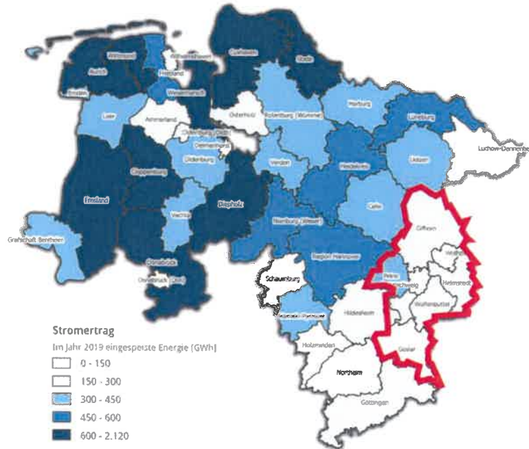
ABBILDUNG 10: STROMERTRAG AUS WINDENERGIEANLAGEN
